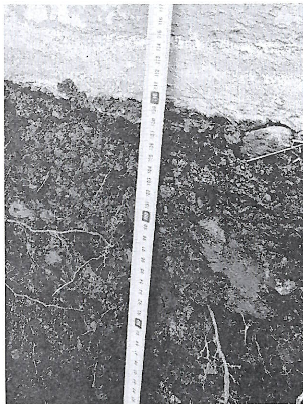
Fig. 10 Dezvelire de fundație realizată la adâncimea de D_f = 1,10 m
