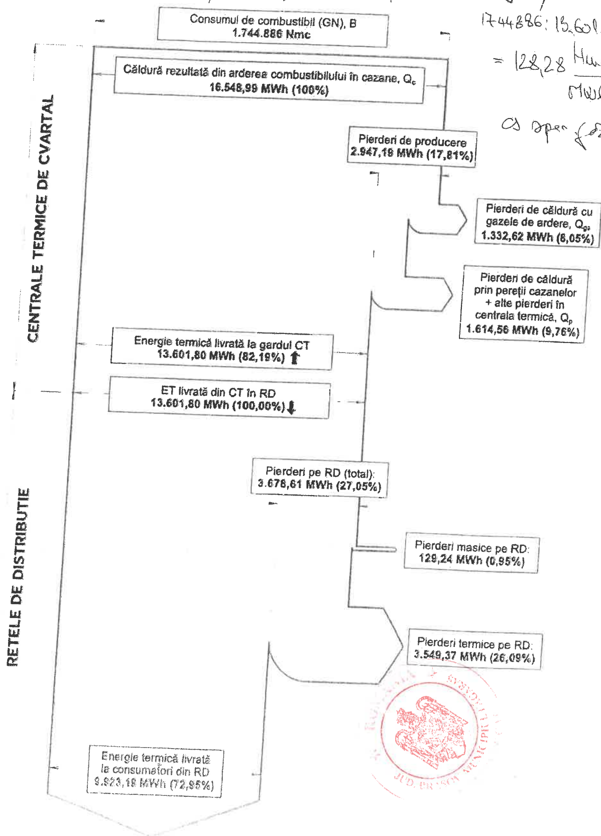
Fig. 3.1. Diagrama Sankey pentru bilanțul real anual al SACEI Făgăraș
