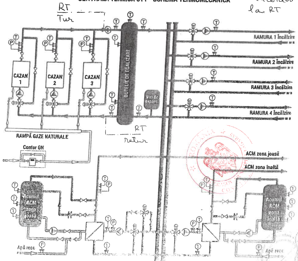
Fig. 2.13. Centrala termică CT1 - schema termomecanică
