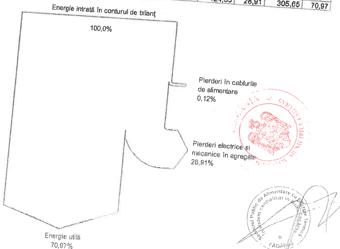
Fig. 8.25. Diagrama Sankey pentru bilanțului electroenergetic ANUAL pe conturul general al auditului
