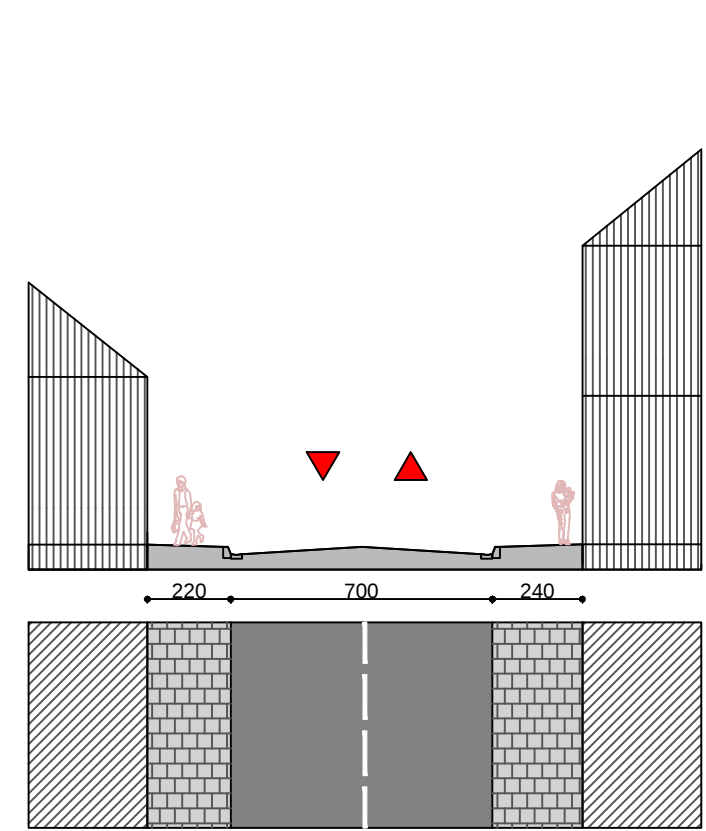
STRADA MIHAI EMINESCU X - X'
