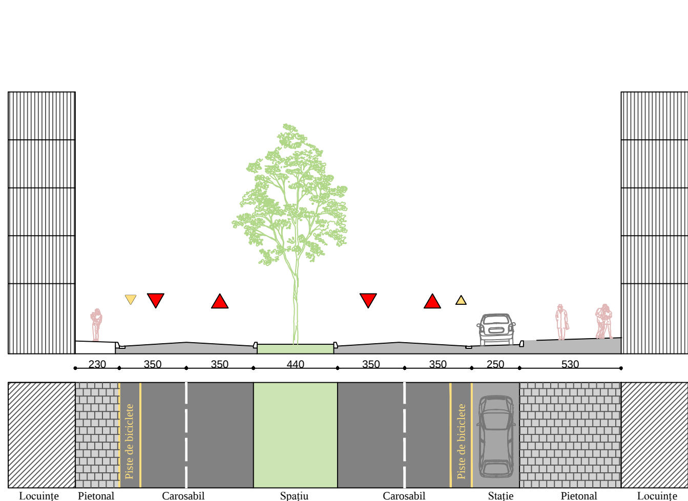
BULEVARDUL UNIRII B - B'
