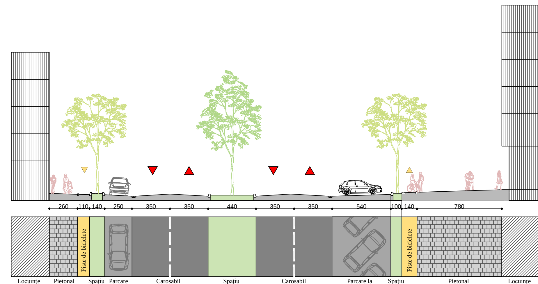
BULEVARDUL UNIRII C - C'
