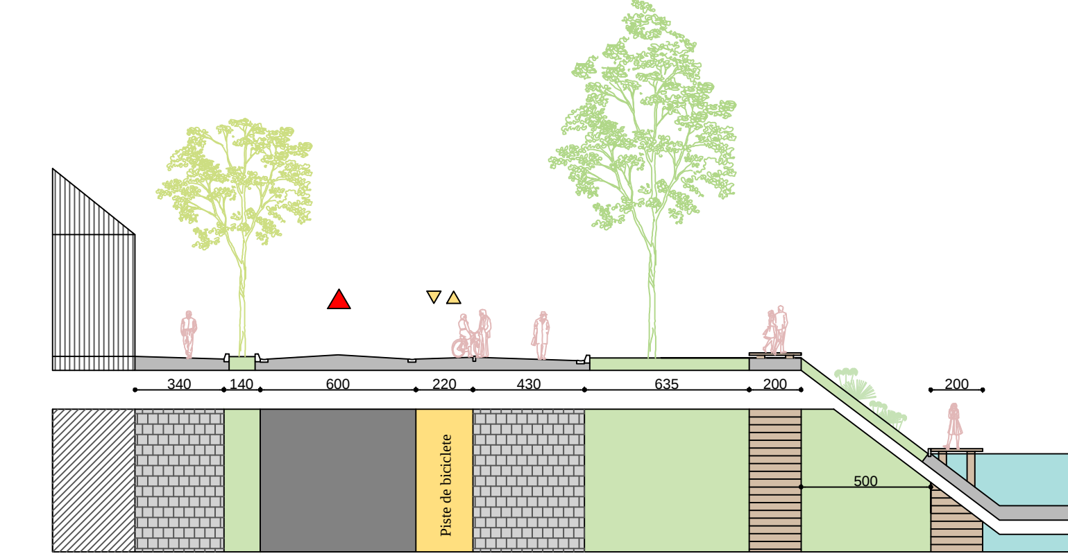
STRADA MIHAI VITEAZUL J - J'
