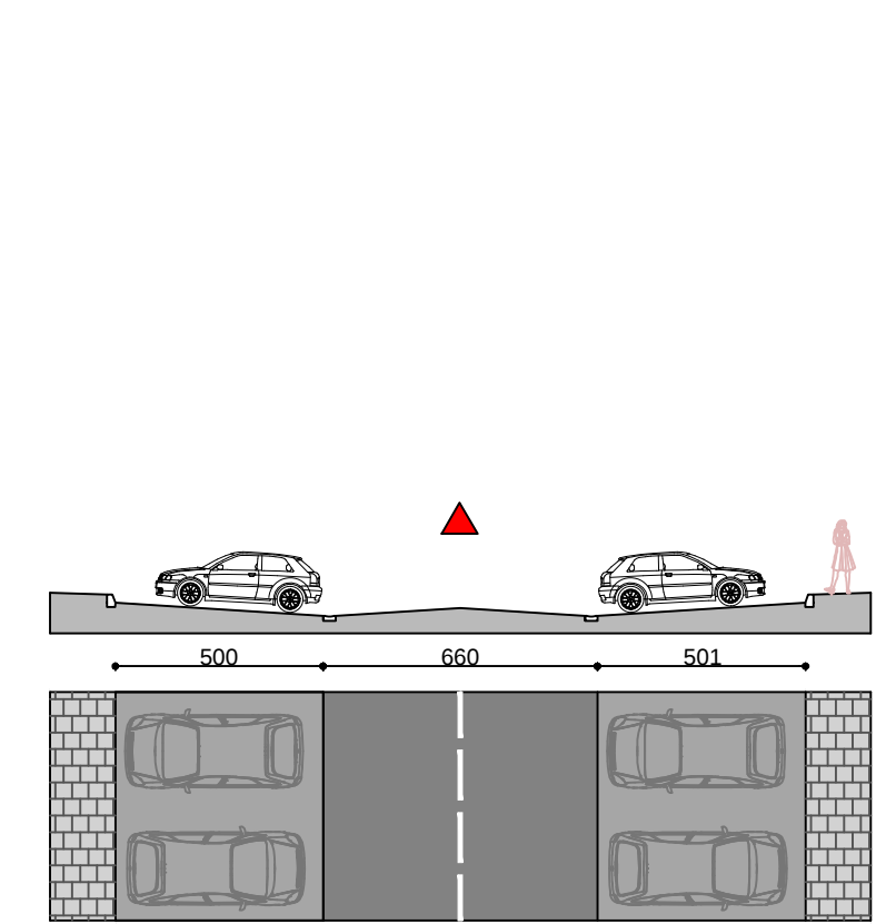
STRADA MIHAI EMINESCU ZONA PIEȚEI Y - Y'
