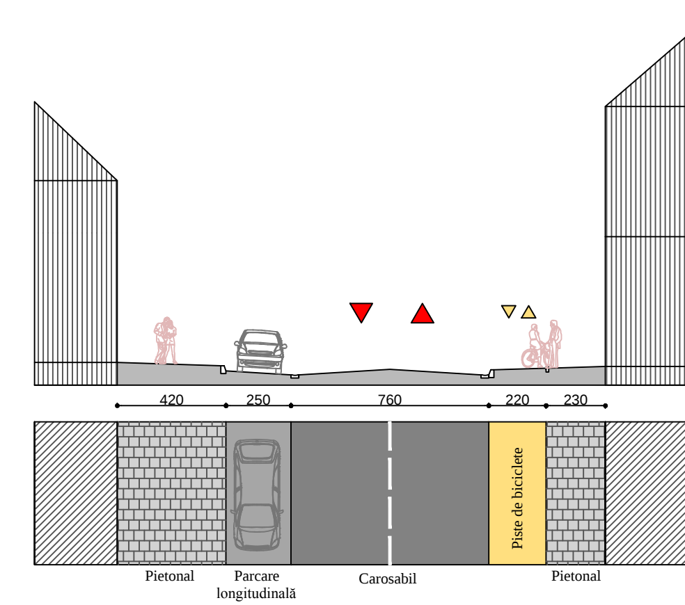
STRADA REPUBLICII O - O'
