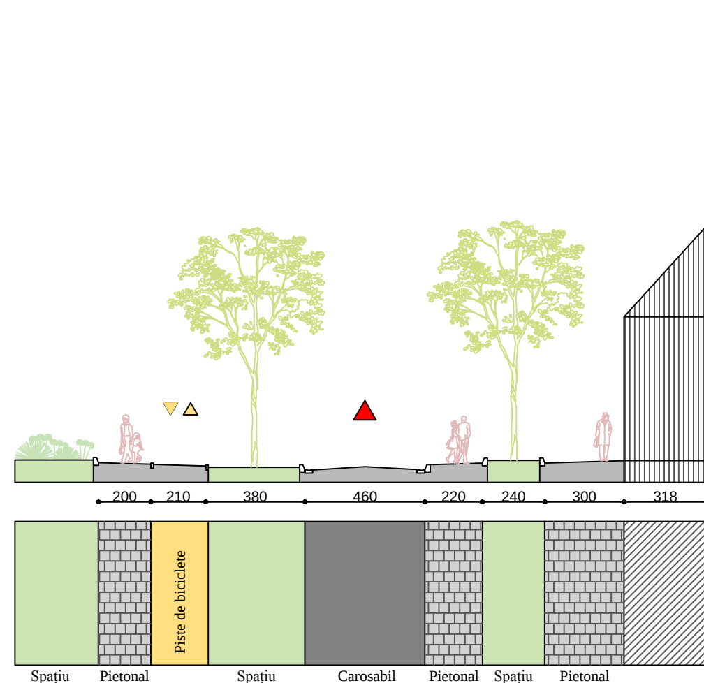
STRADA DOAMNA STANCA D - D'
