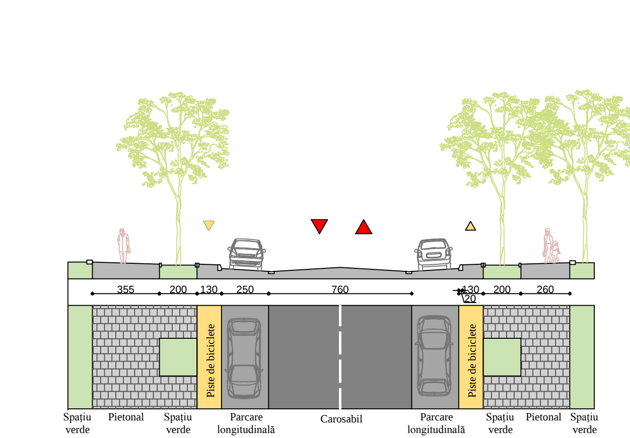
STRADA MIHAI VITEAZUL M - M'
