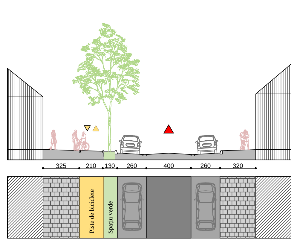
STRADA DOAMNA STANCA F - F'
