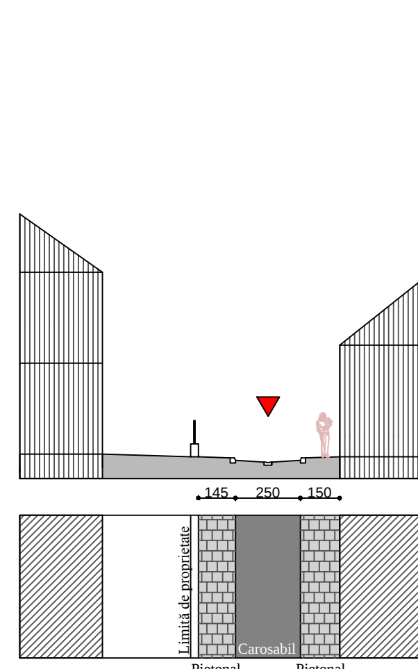
STRADA GH. BARIȚIU DD - DD'
