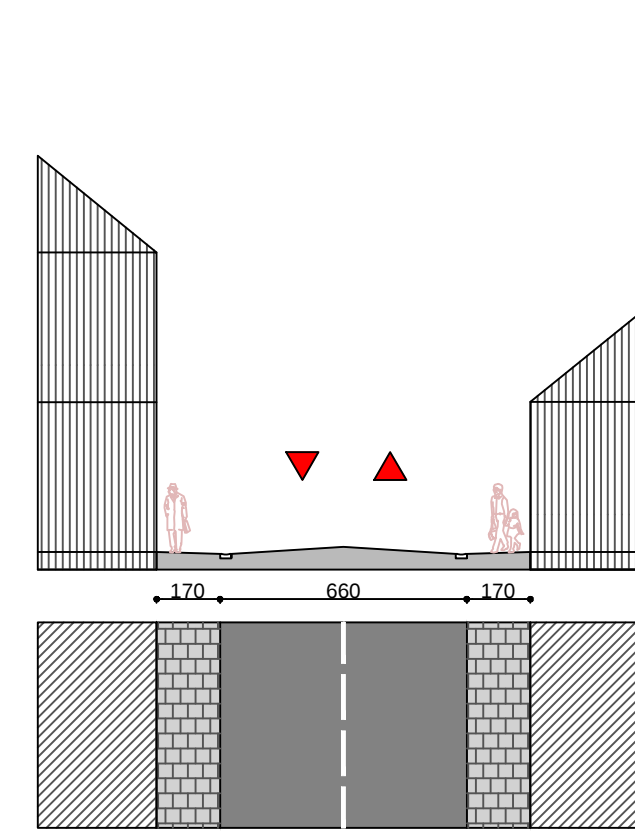
STRADA I.M. KLEIN/ TITU PERȚIA S - S'
