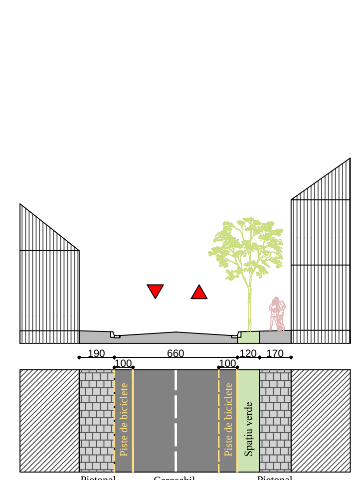
STRADA PODULUI EE - EE'
