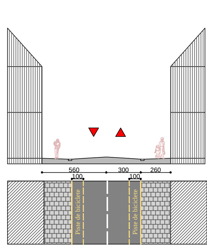
STRADA DOAMNA STANCA G - G'
