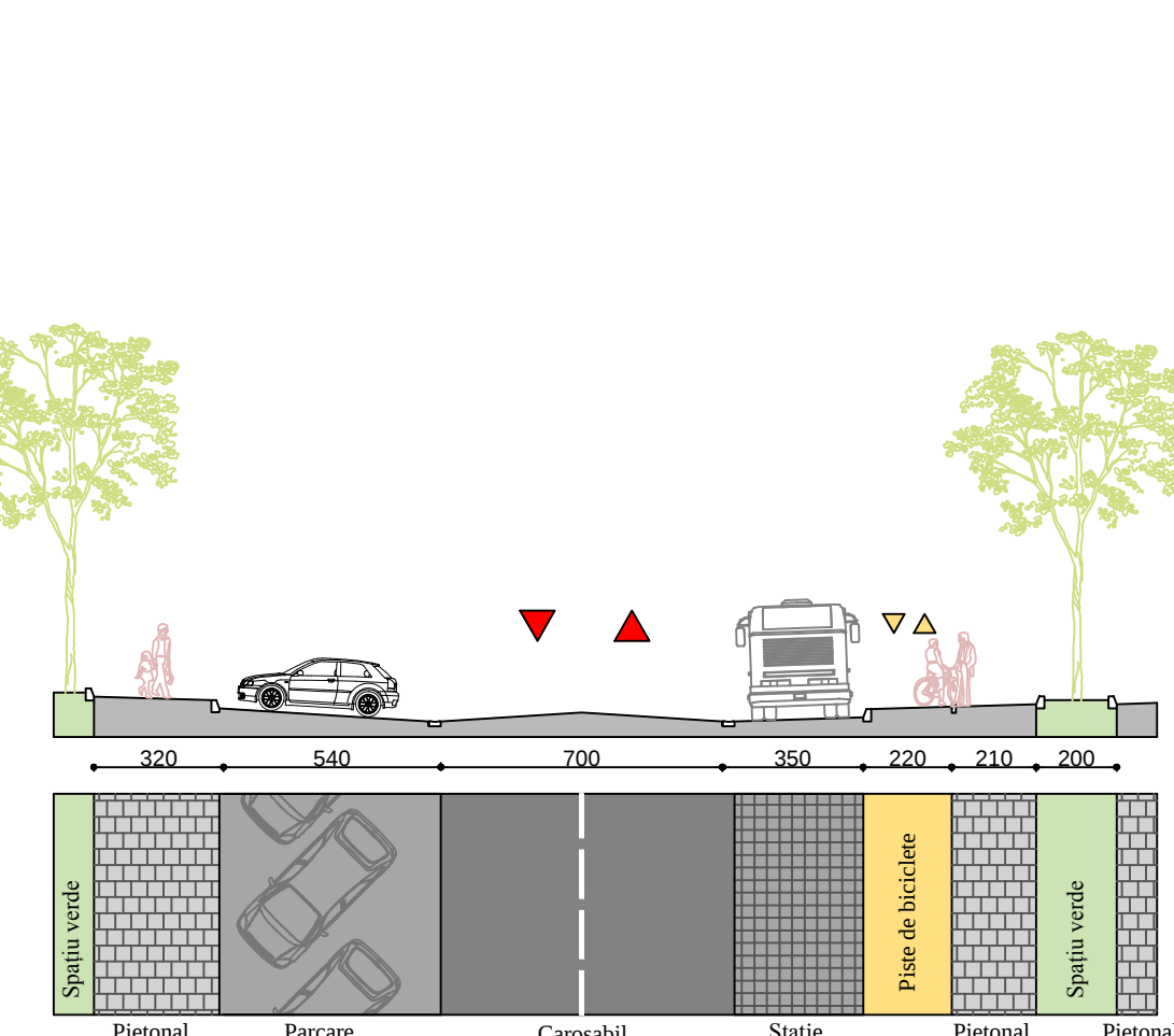
STRADA TEIULUI BB - BB'
