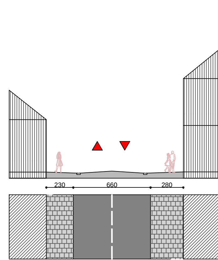
STRADA TITU PERȚIA T - T'
