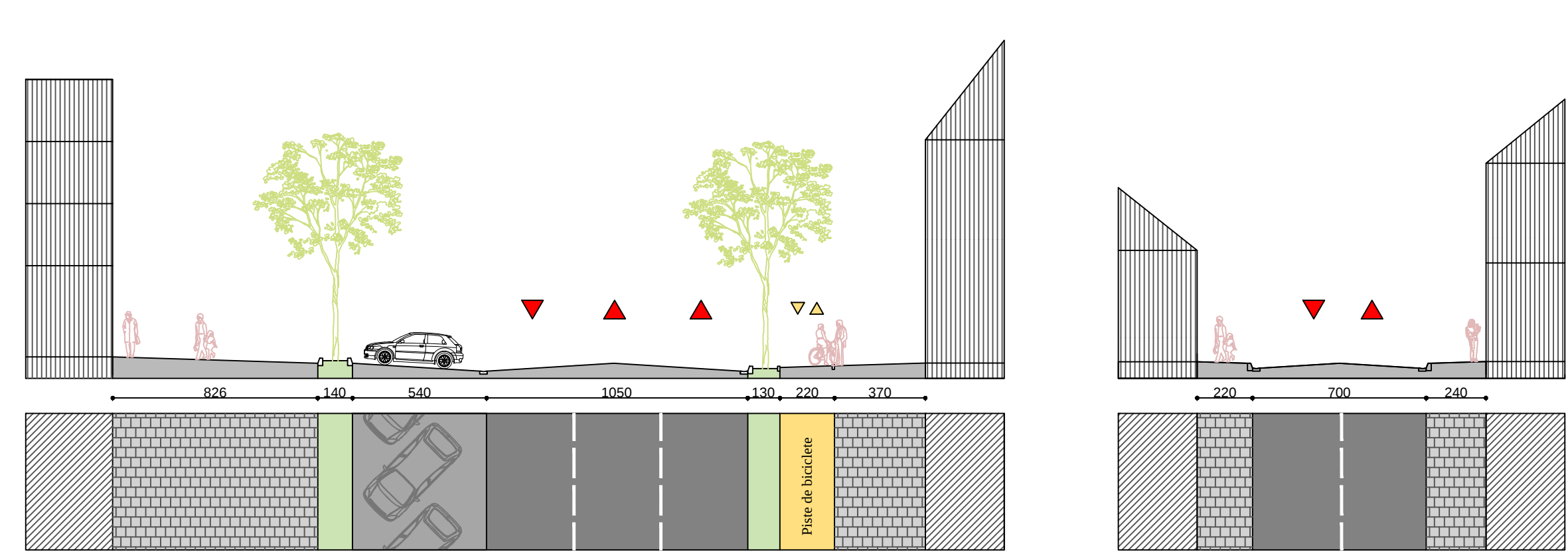
STRADA MIHAI EMINESCU W - W'
