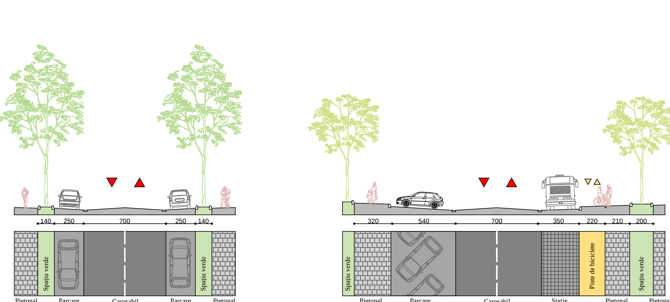
STRADA 1 DECEMBRIE AA - AA'
