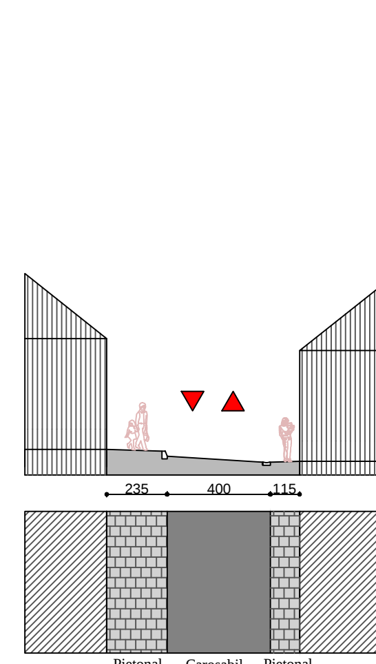
STRADA CETĂȚII FF - FF'
