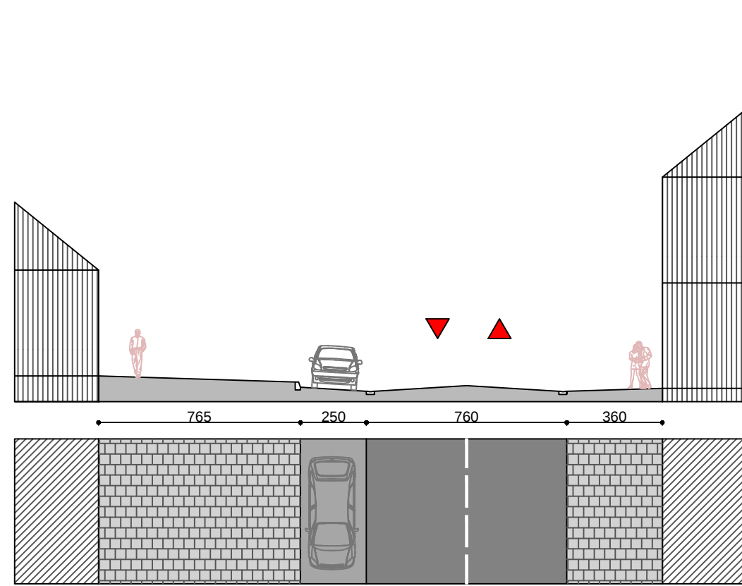
STRADA LIBERTĂȚII R - R'
