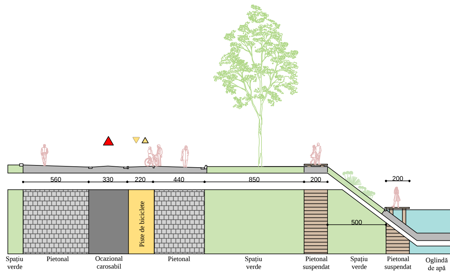
STRADA MIHAI VITEAZUL K - K'
