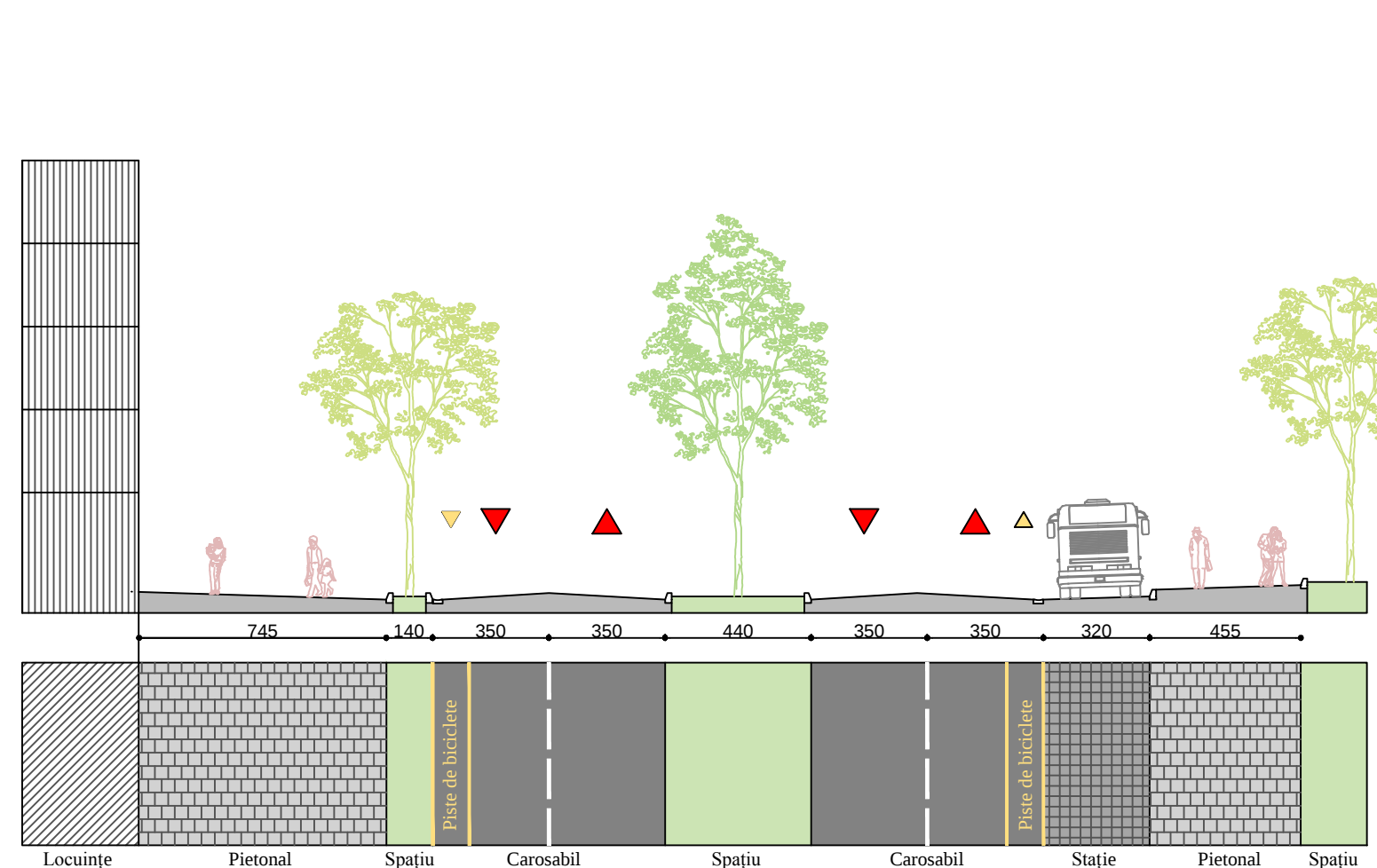
BULEVARDUL UNIRII A - A'
