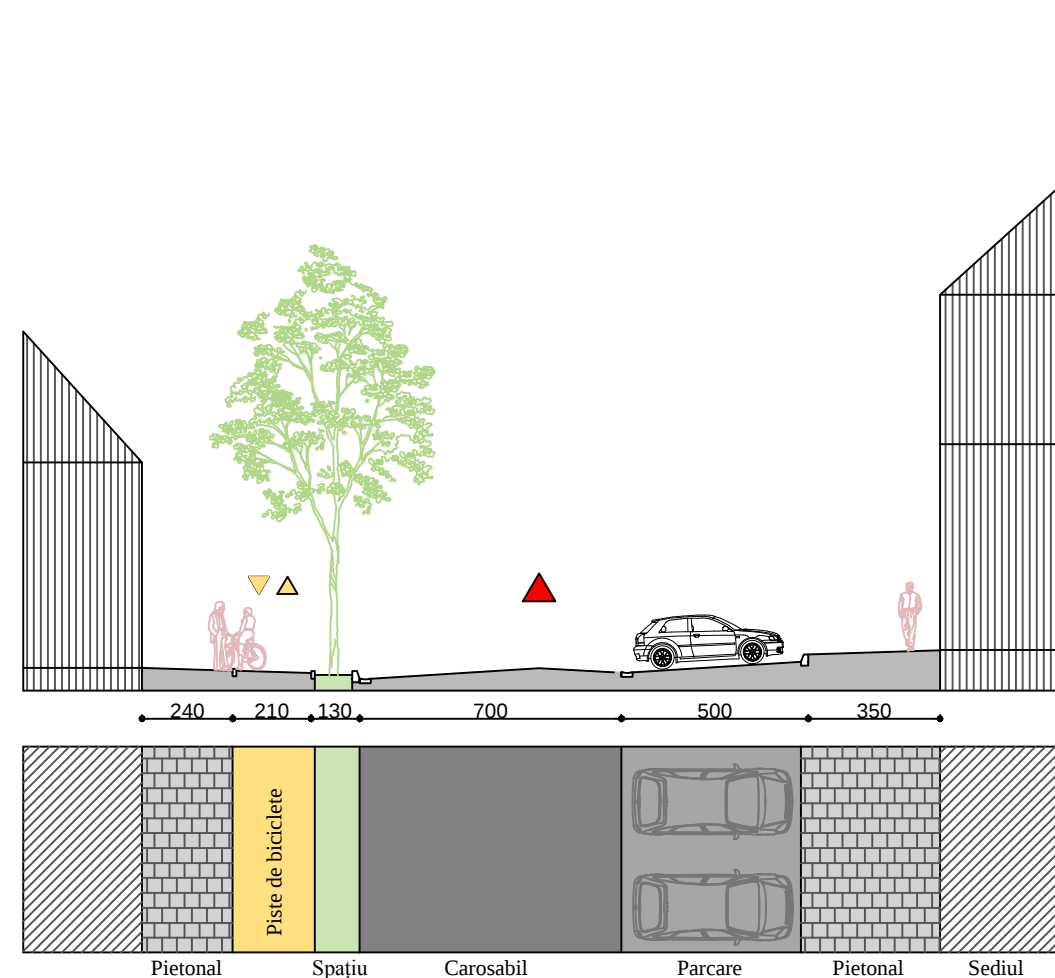
STRADA DOAMNA STANCA E - E'
