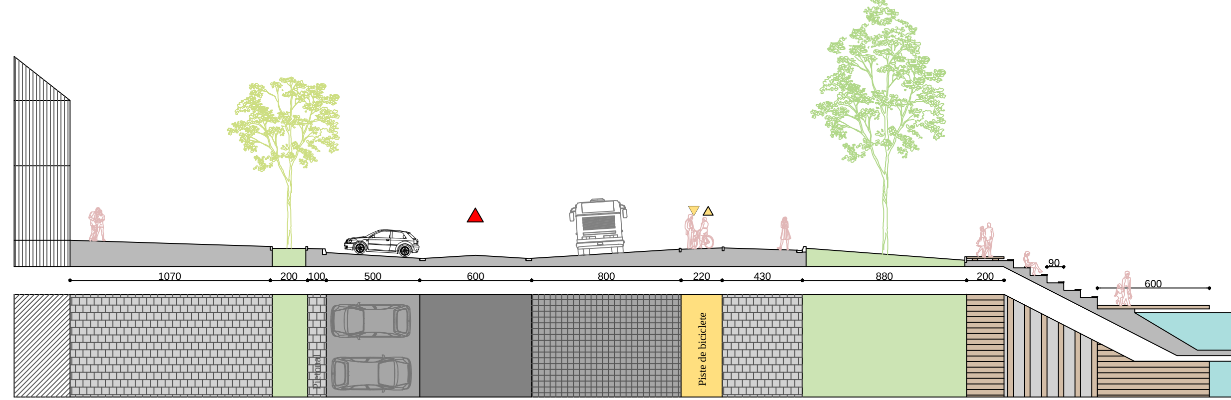
STRADA MIHAI VITEAZUL I - I'
