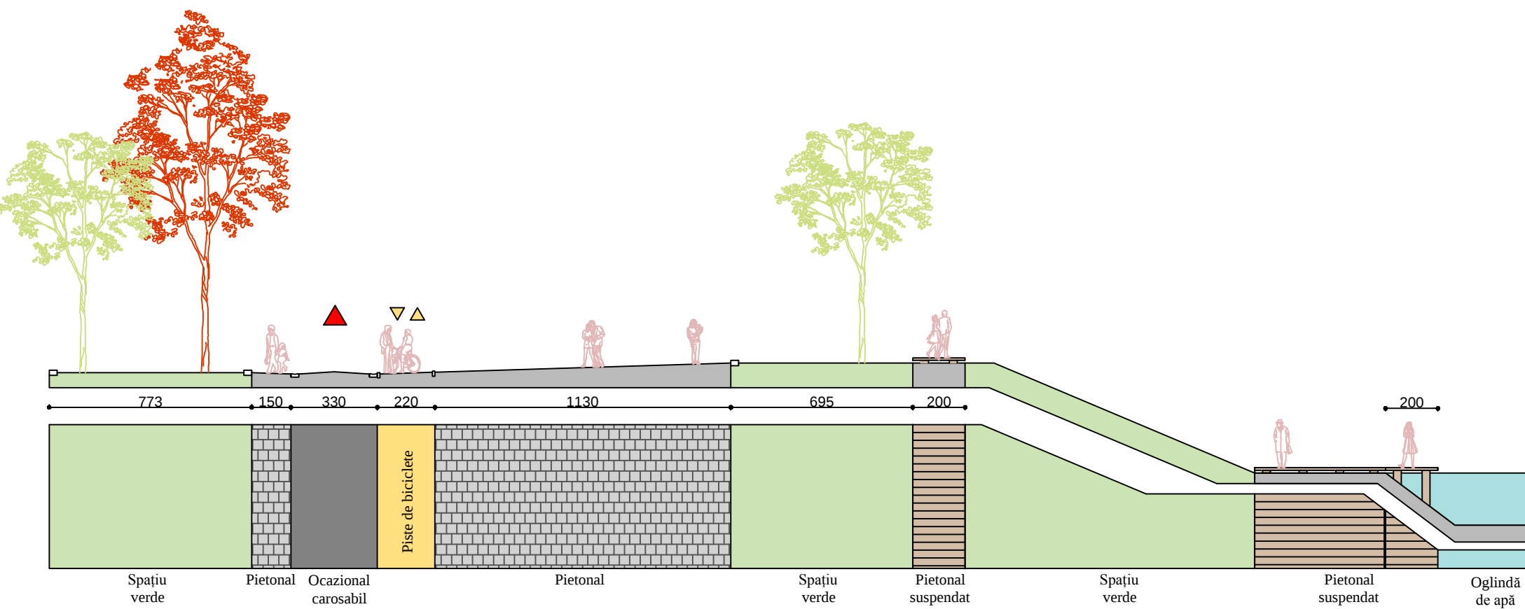
STRADA MIHAI VITEAZUL L - L'
