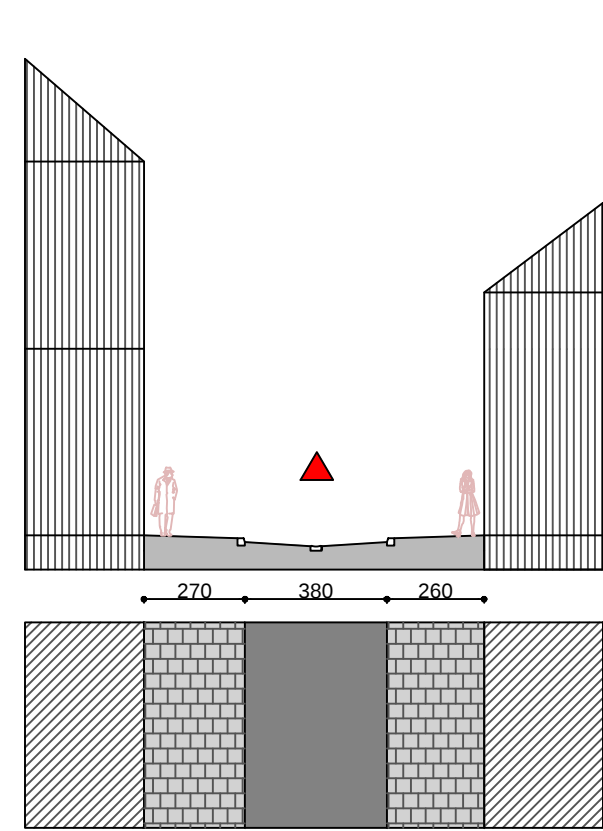
STRADA I. C. DRĂGUȘANU /CONSTANTIN POPP Q - Q'
