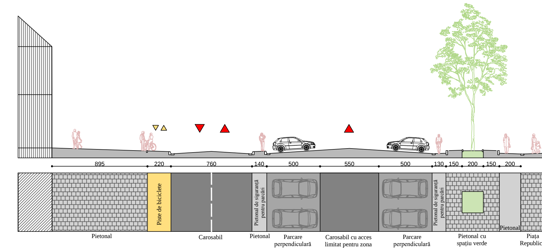
STRADA REPUBLICII N - N'
