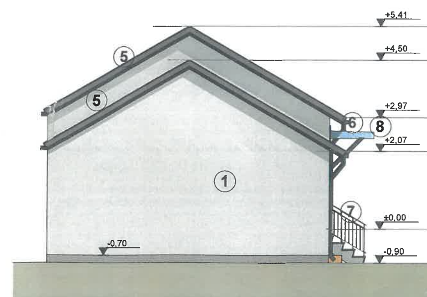
FATADA SUD LOCUINTA PROPUNERESC.1:100
