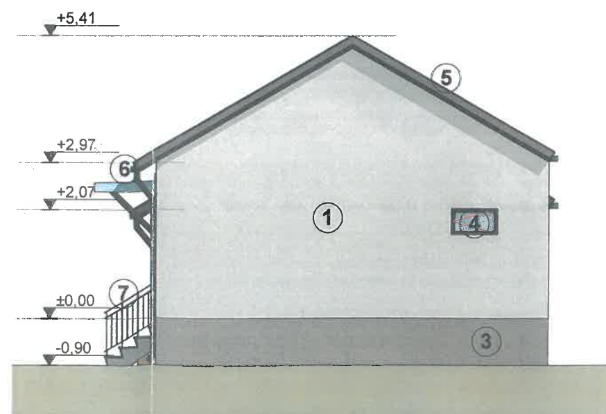
FATADA NORD LOCUINTA PROPUNERESC.1:100
