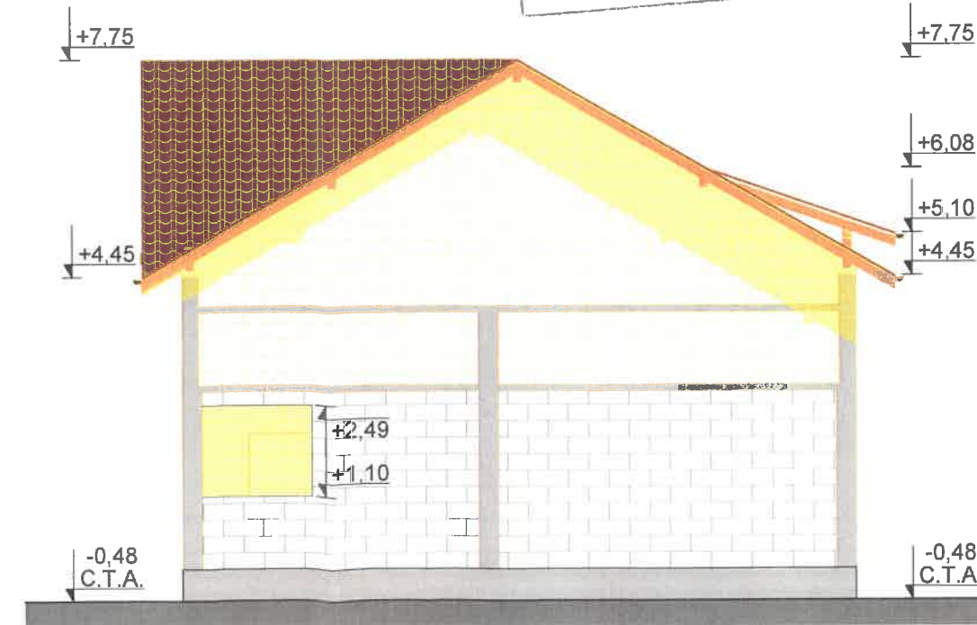
FAȚADA EST - RELEVU scara 1:100, 1:50
