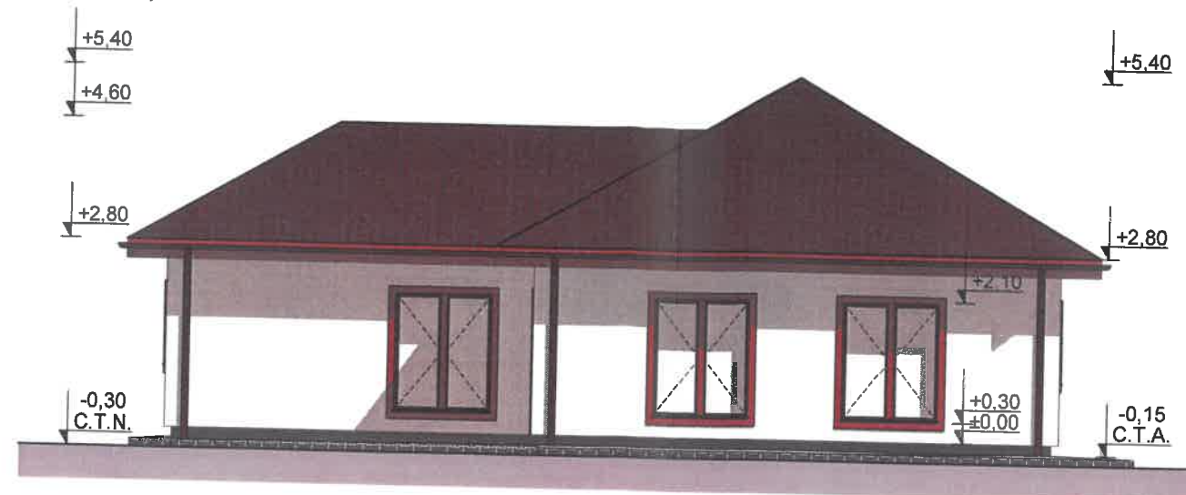
FAȚADA SUD scara 1:100, 1:50
