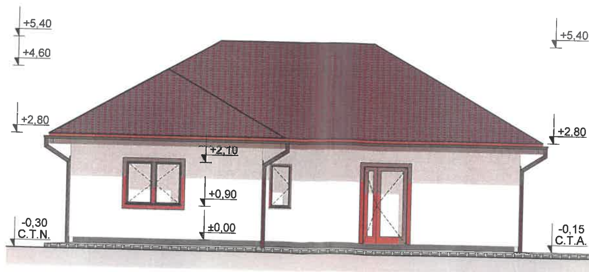
FAȚADA VEST scara 1:100, 1:50
