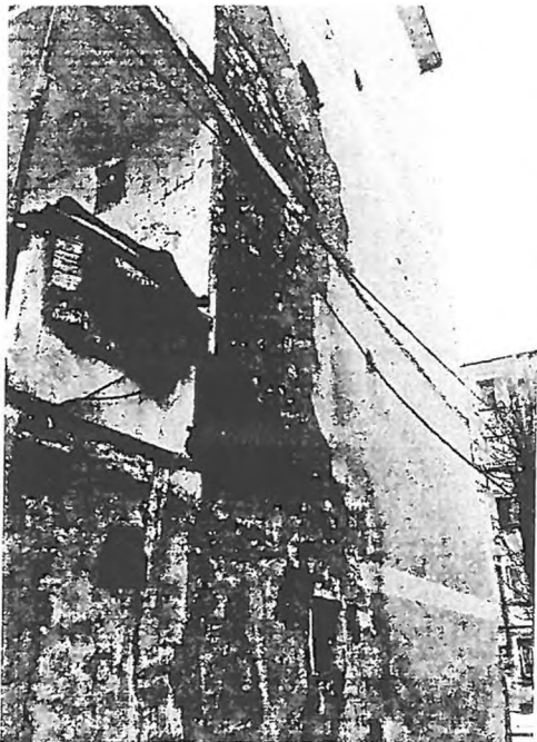
Degradarea parții de rezistență
