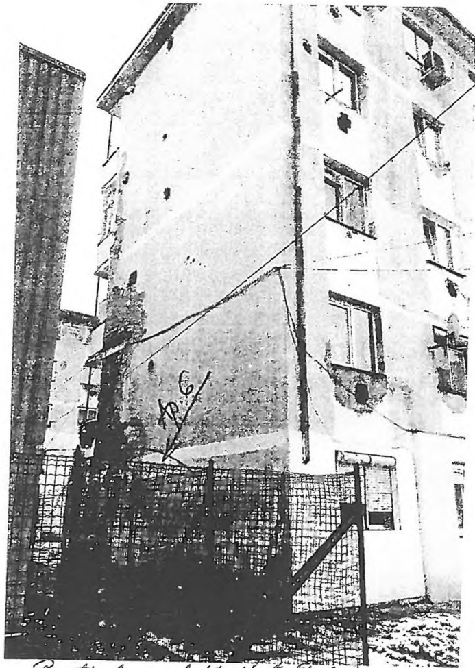
Pereti degradati afectati de igrosie
