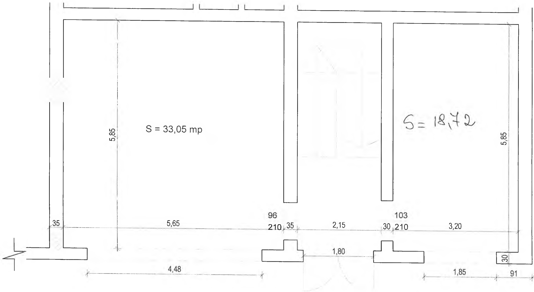
RELEVU SCARA 1 : 50
